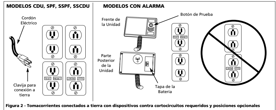
Figura 2 - Tomacorrientes conectados a tierra con dispositivos contra cortocircuitos requeridos y posiciones opcionales
